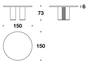
TTV (40E) - TTV (40M) TAVOLO / TABLE Ø 150x73H. - THK.6cm Ø 59x28 2/3H. - THK.2 6/16"
