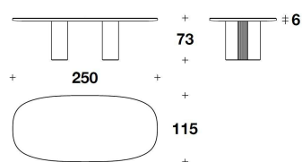
TTV (37E) - TTV (37M) TAVOLO / TABLE 250x115x73H. - THK.6cm 98 1/3x45 1/3x28 2/3H. - THK.2 6/16"
