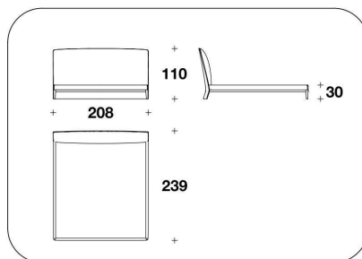
NWE (KUSA) KING USA : LETTO PER MATERASSO / BED FOR MATTRESS 195x205 - 208x239x110H. - H.B.30cm 76 2/3x80 2/3 - 82x94x43 1/3H. - H.B.11 3/4"
