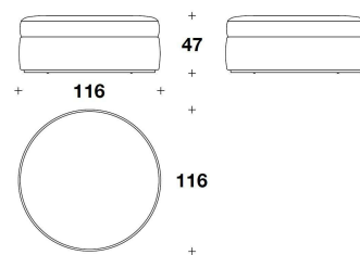
PUP (POUG) BIG : POUF / OTTOMAN Ø 116x47H.cm Ø 45 2/3x18 2/4H."
