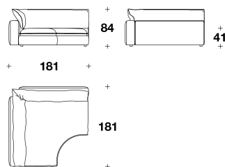
SOT (ANG) ELEMENTO ANGOLARE / CORNER ELEMENT 181x181x84H. - H.S.41cm 71 1/3x71 1/3x33H. - H.S.16 1/4"
