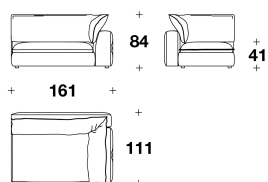
SOT (E1XD) - SOT (E1XS) MAXI : ELEMENTO CON BRACCIOLO DX O SX / ELEMENT WITH RIGHT OR LEFT ARMREST 161x111x84H. - H.S.41cm 63 1/3x4 1/4x33H. - H.S.16 1/4"
