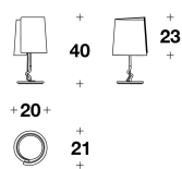
TRL (34) LAMPADA DA TAVOLO NOTTE / BEDSIDE TABLE LAMP 20x21x40H.cm 7 3/4x8 1/4x15 3/4H."
