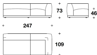
1BL (E3AD) - 1BL (E3AS) ELEMENTO ANGOLARE 3 POSTI CON ANGOLO DX O SX / 3 SEATER CORNER ELEMENT WITH RIGHT OR LEFT CORNER 247x109x73H. - H.S.46cm 97 1/3x43x28 2/3H. - H.S.18"
