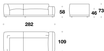
1BL (D3AD) - 1BL (D3AS) DIVANO ANGOLARE 3 POSTI CON BRACCIOLO DX O SX / 3 SEATER CORNER SOFA WITH RIGHT OR LEFT ARMREST 282x109x73H. - H.S.46cm 111x43x28 2/3H. - H.S.18"
