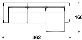
SQU (E3S) + SQU (CLD) A) : ESEMPIO DI COMPOSIZIONE / SECTIONAL SOFA EXAMPLE 362x160x88H. - H.S.44cm 142 1/2x63x34 2/3H. - H.S.17 1/4"
