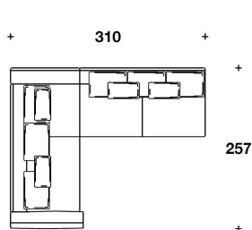
ELN (AD1AS) + ELN (AE2C) E) : ESEMPIO DI COMPOSIZIONE / SECTIONAL SOFA EXAMPLE 310x257x98H. - H.S.47cm 122x101 1/3x38 2/3H. - H.S.18 2/4"
