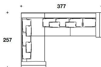
ELN (AD1AS) + ELN (AE4D) L) : ESEMPIO DI COMPOSIZIONE / SECTIONAL SOFA EXAMPLE 377x257x98H. - H.S.47cm 148 1/2x101 1/3x38 2/3H. - H.S.18 2/4"
