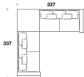
ELN (AE2S) + ELN (POUQ) + ELN (AE2D) G) : ESEMPIO DI COMPOSIZIONE / SECTIONAL SOFA EXAMPLE 337x337x98H. - H.S.47cm 132 2/3x132 2/3x38 2/3H. - H.S.18 2/4"
