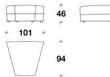
DLS (POUT) TRAPEZIUM : POUF / OTTOMAN 101x94 - H.S.46cm 39 2/3x37 - H.S.18"
