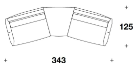
DLS (EGS) + DLS (POUT) + DLS (EGD) A) : ESEMPIO DI COMPOSIZIONE / SECTIONAL SOFA EXAMPLE 343x125x81H. - H.S.46cm
