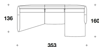
DLS (EOS) + DLS (ECP) + DLS (CLD) C) : ESEMPIO DI COMPOSIZIONE / SECTIONAL SOFA EXAMPLE 353x160x81H. - H.S.46cm
