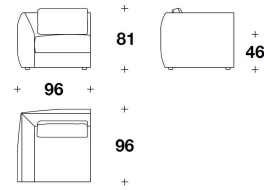
DLS (ANG) ELEMENTO ANGOLARE QUADRATO / SQUARE CORNER ELEMENT 96x96x81H. - H.S.46cm 37 2/3x37 2/3x32H. - H.S.18"
