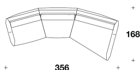
DLS (EPS) + DLS (CNT) + DLS (EOD) B) : ESEMPIO DI COMPOSIZIONE / SECTIONAL SOFA EXAMPLE 356x168x81H. - H.S.46cm
