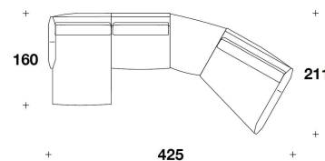
DLS (CLS) + DLS (ECP) + DLS (POUT) + DLS (EOD) F) : ESEMPIO DI COMPOSIZIONE / SECTIONAL SOFA EXAMPLE 425x211x81H. - H.S.46cm
